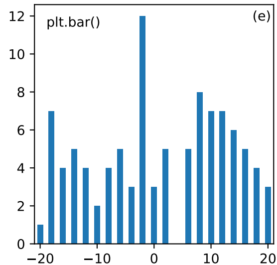
numpy.unique
